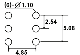
C - DPDT
