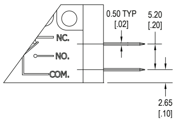
SPST N.O.
