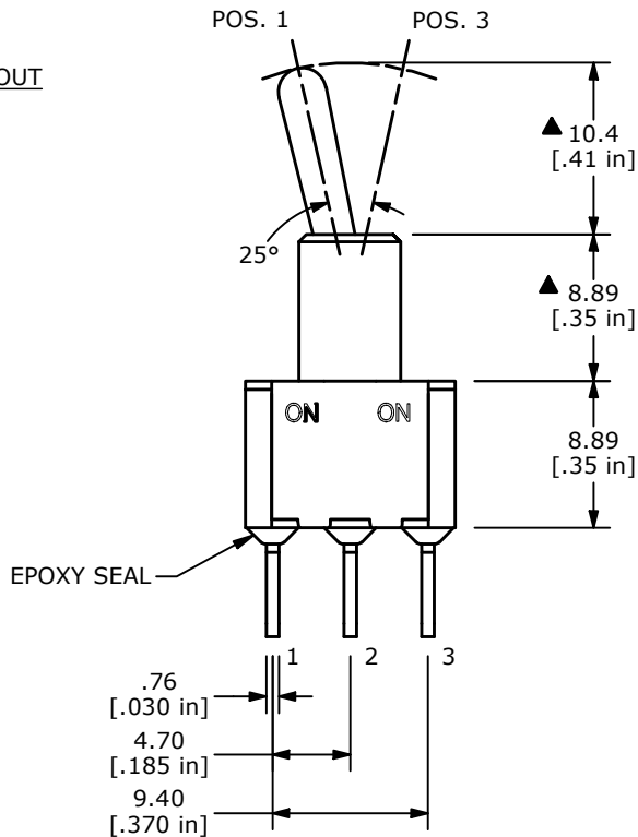
CIRCUIT: SPDT
