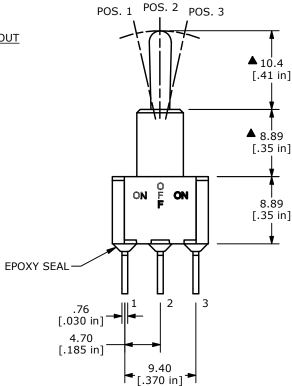
CIRCUIT: SPDT
