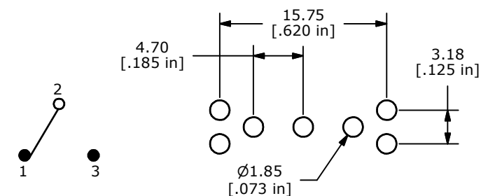
CIRCUIT: SPDT
