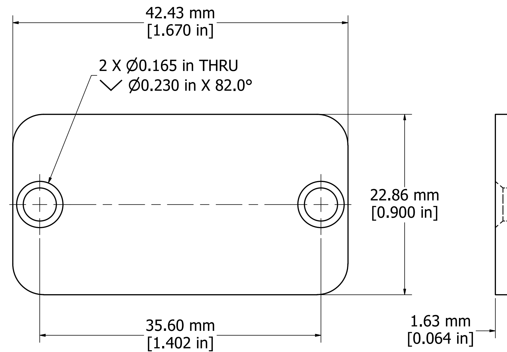
ENDPLATE
