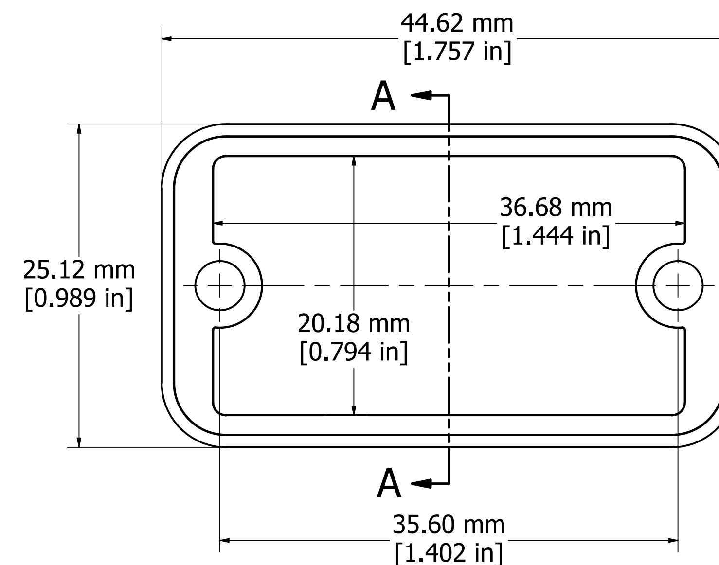
OPEN BEZEL
