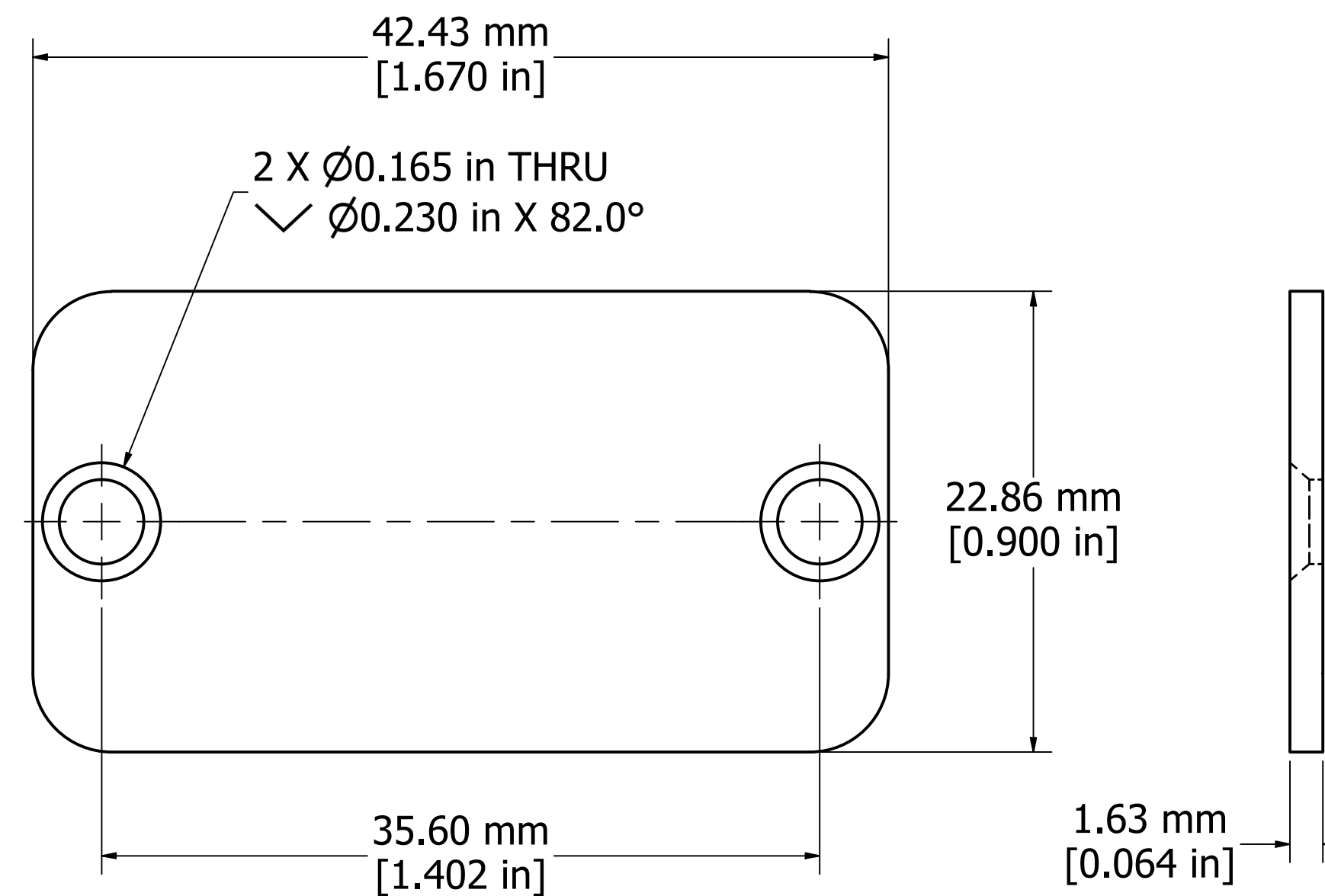
ENDPLATE
