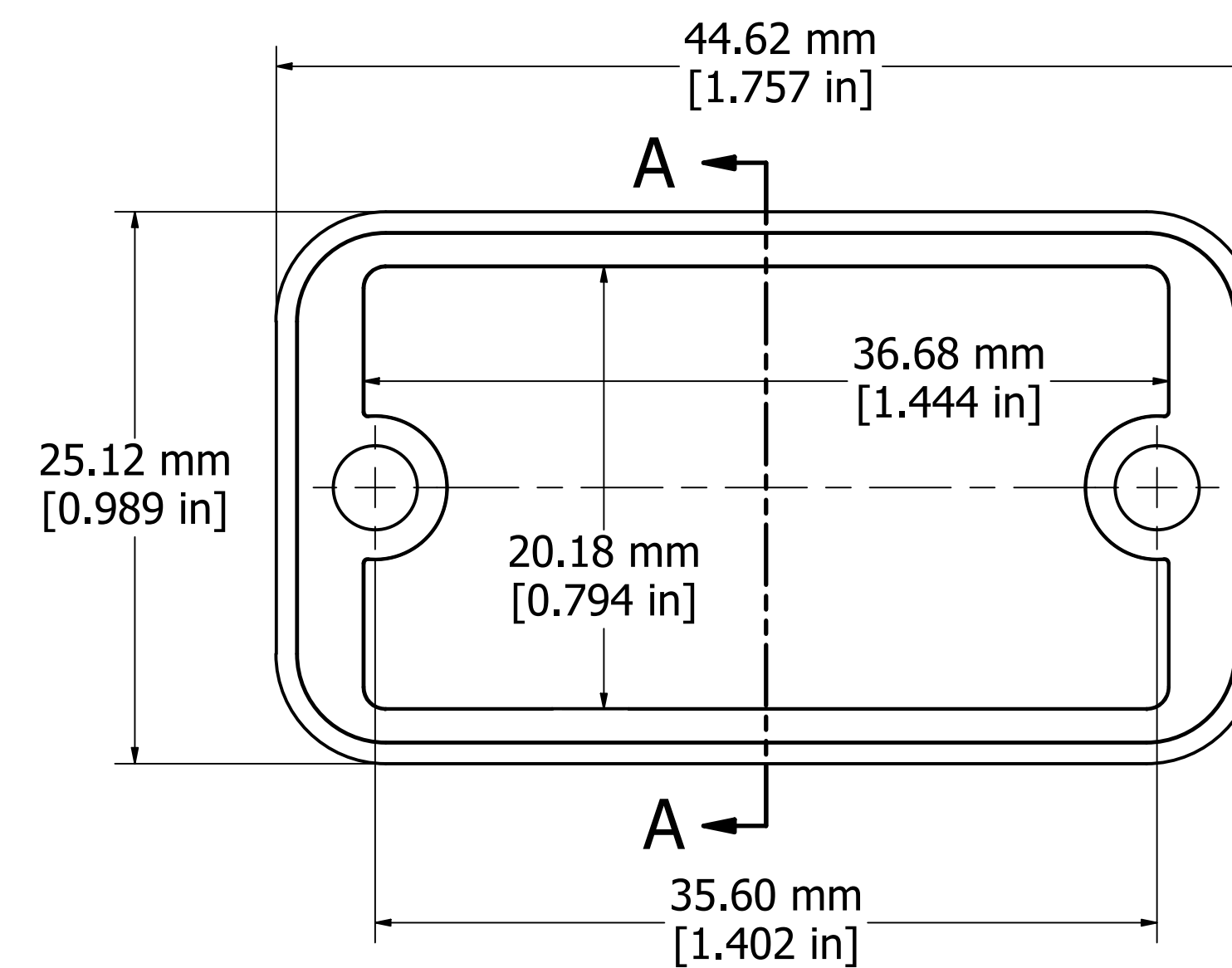
OPEN BEZEL
