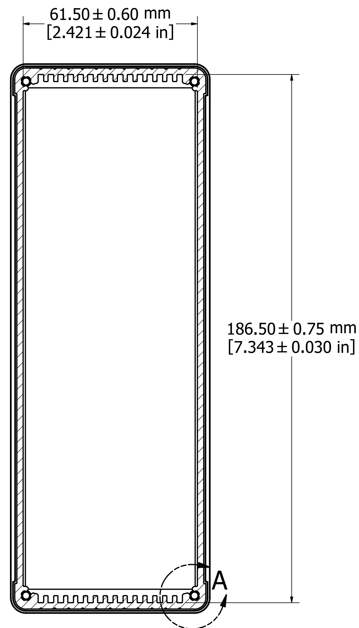
SECTION A-A
