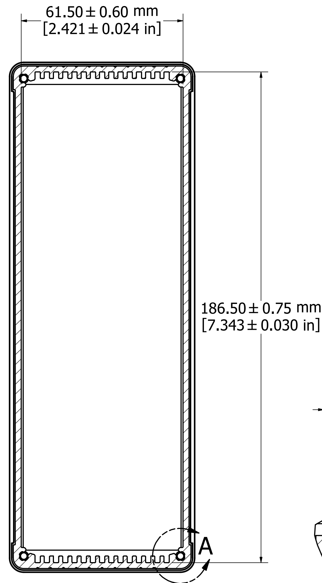
SECTION A-A
