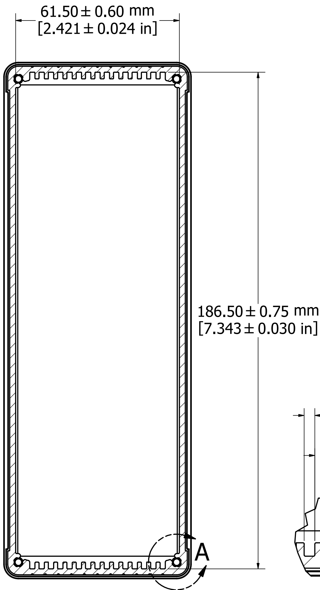
SECTION A-A
