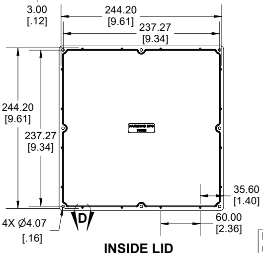
INSIDE LID
