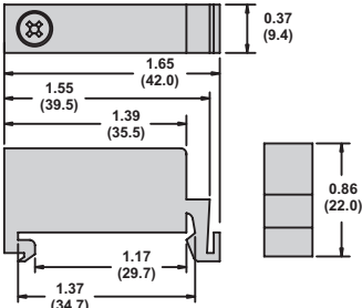
16-DCLIP-1 DIN Rail End Clip
