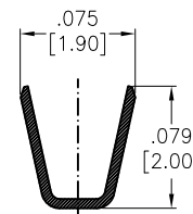
SECTION D-D
