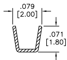
A-A SEC.
