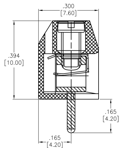
SECTION A-A
